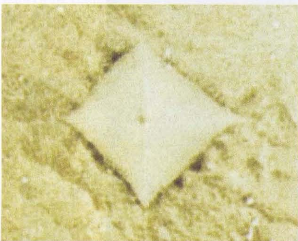
Figura 7: huella de indentación
