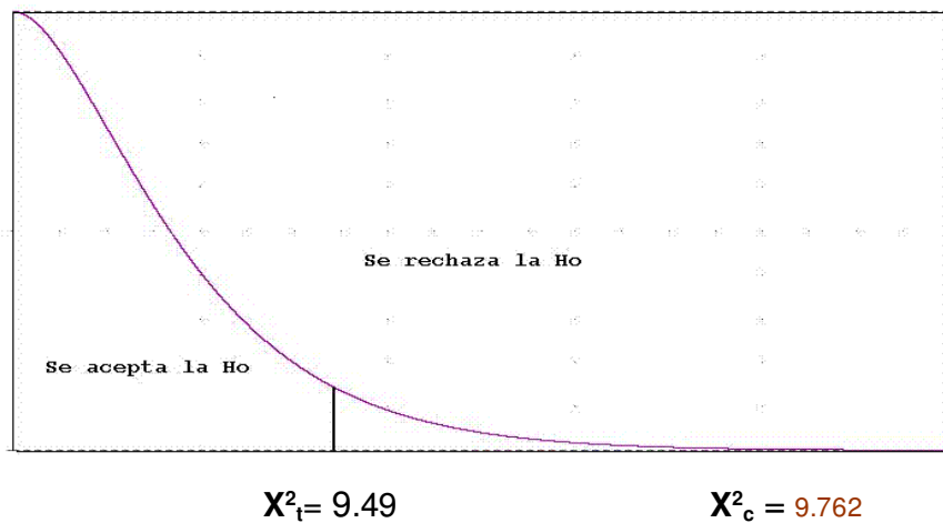
Figura 19. Prueba de Chi-cuadrado
