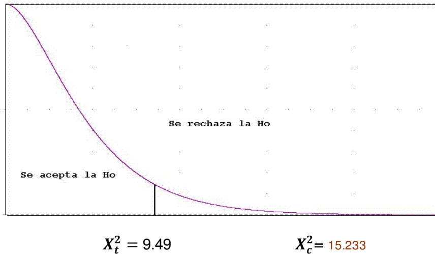
Figura 15. Prueba de Chi-cuadrado
