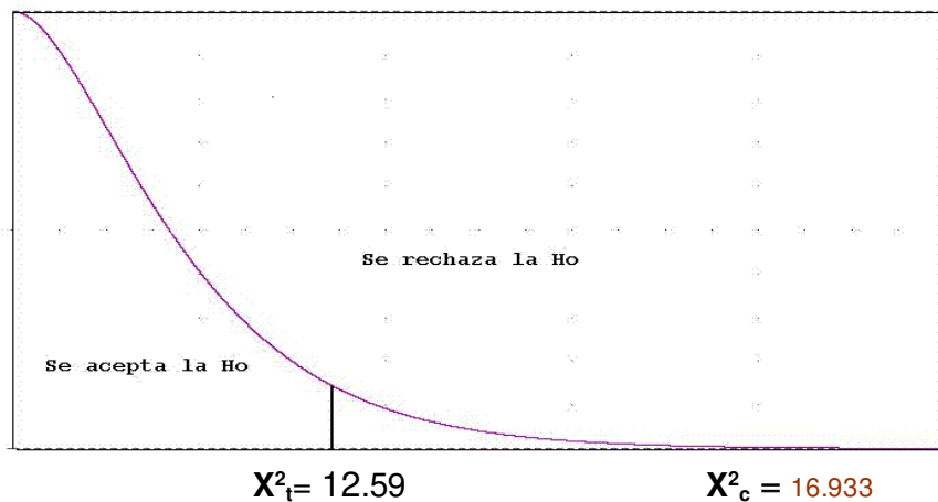
Figura 17. Prueba de Chi-cuadrado
