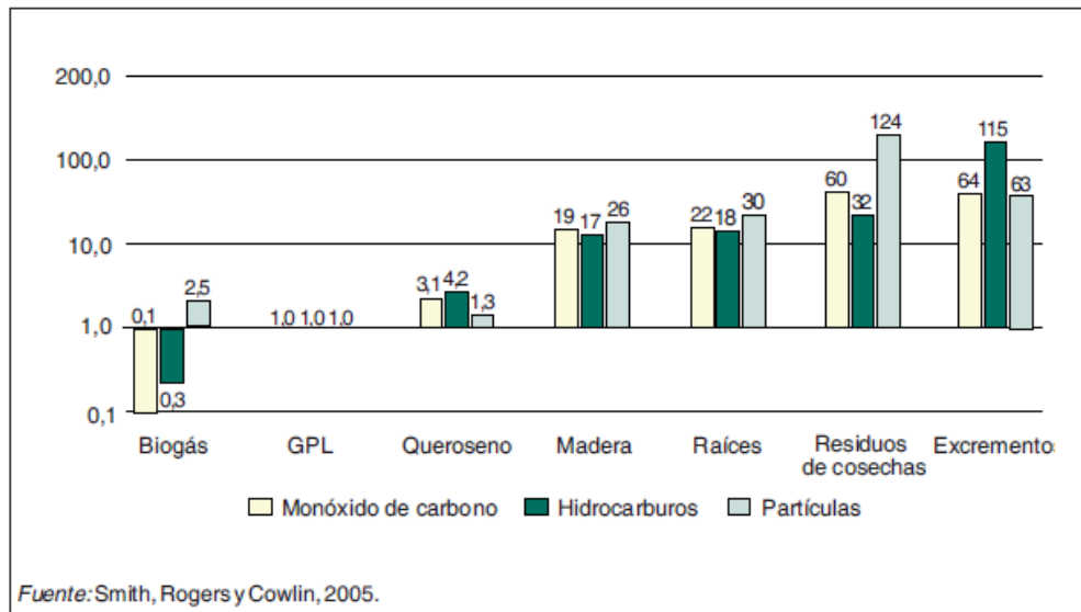
Figura 2. Escala de la energía: emisiones contaminantes por comida según el combustible utilizado, en relación con el GPL (1,0 en la escala) (medición hecha en la India) (Smith, 2006).
