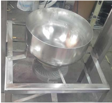
Figura 4. Soporte de olla. Fuente: Elaboración propia.
