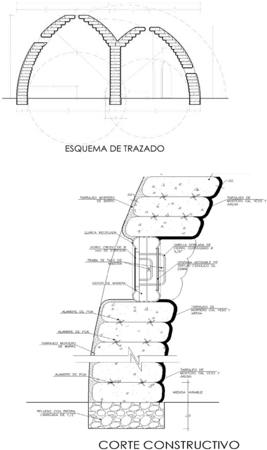
Figura 24. Plano: esquema y detalles constructivos
