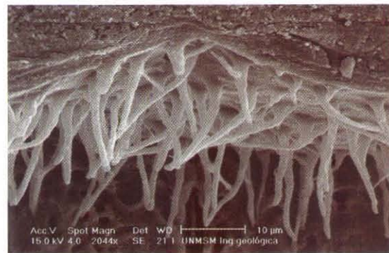
Microfotografía 3. Penetración del agente adhesivo con solvente basado en Etanol. (2004X)
