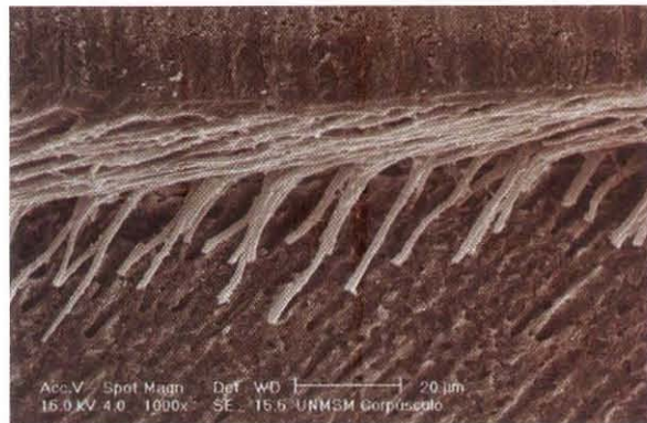
Microfotografía 4: Penetración del agente adhesivo con solvente basado en Acetona. (1000X)
