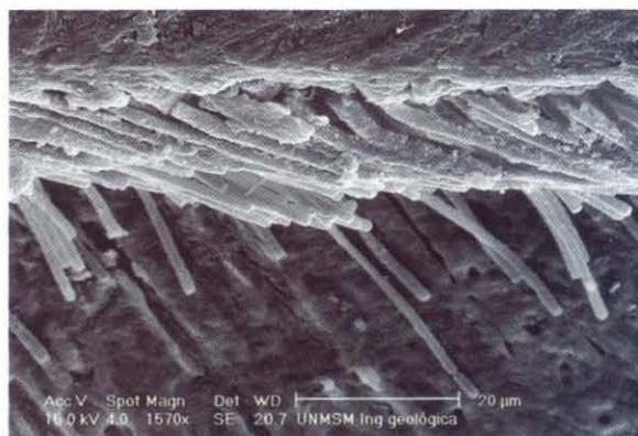
Microfotografía 8: Penetración del agente adhesivo con solvente basado en agua. (1570X)
