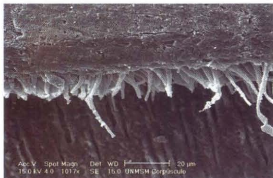
Microfotografía 6: Penetración del agente adhesivo con solvente basado en Acetona. (1017X)
